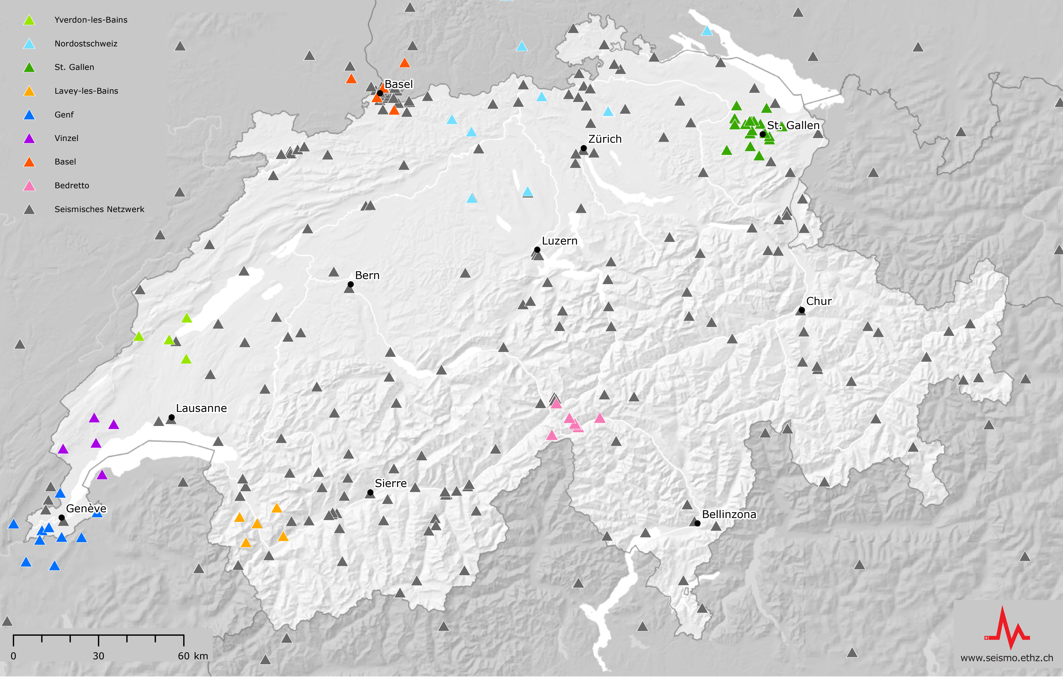
Seismisches Netzwerk der Schweiz mit Spezialnetzwerken
