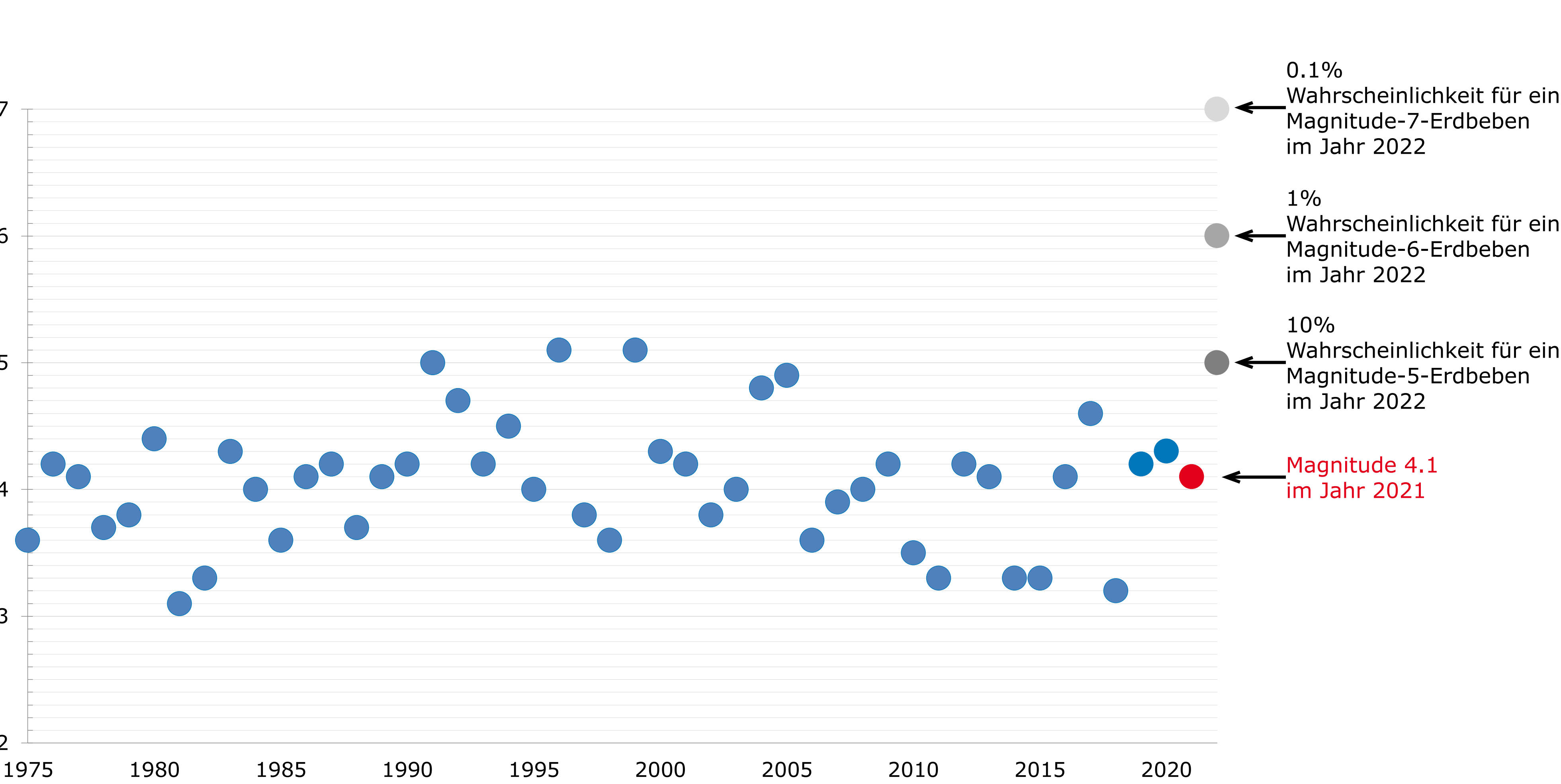
Grösste gemessene Magnitude (M) pro Jahr
