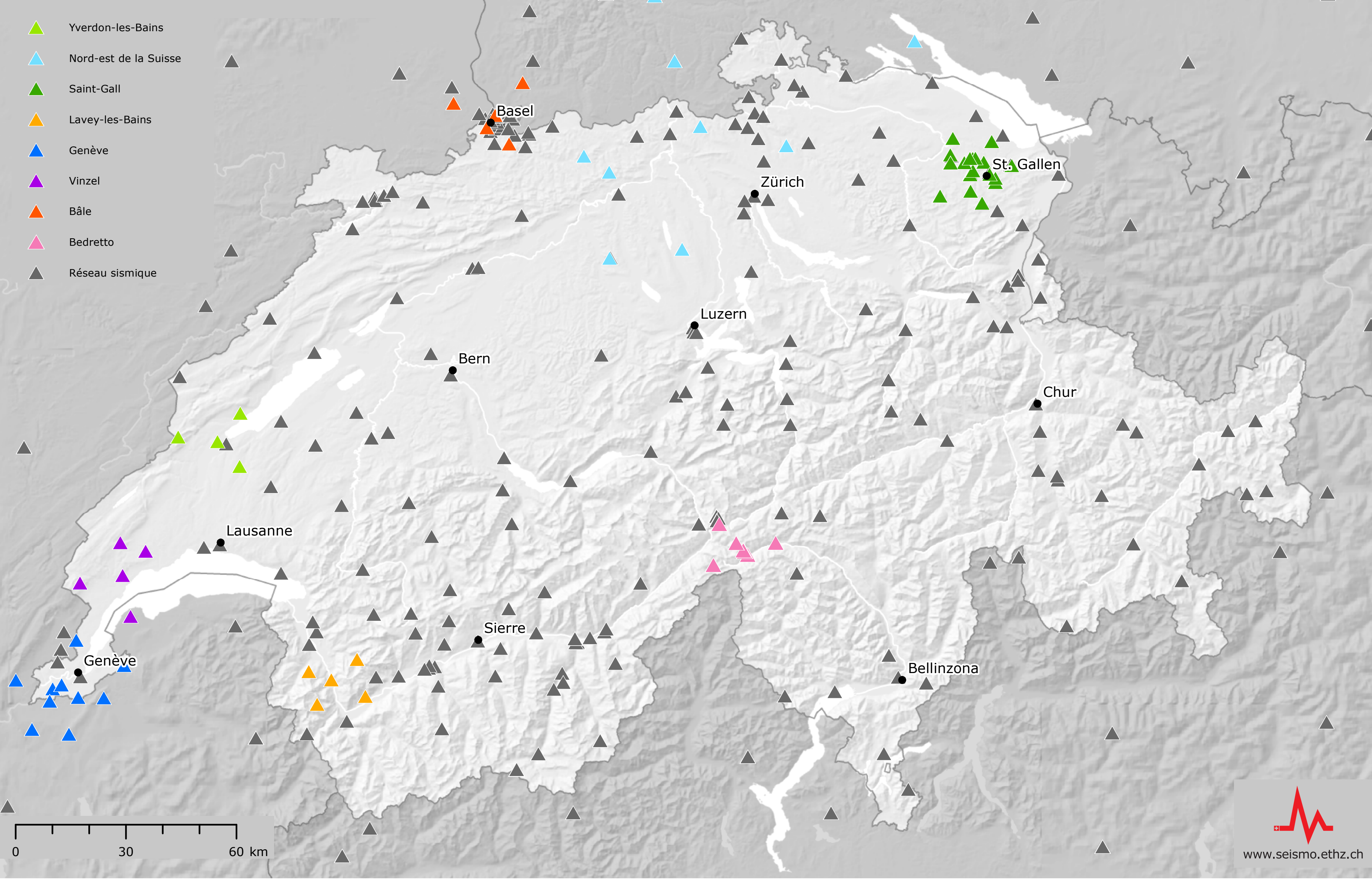
Réseau sismique suisse avec réseaux spéciaux
