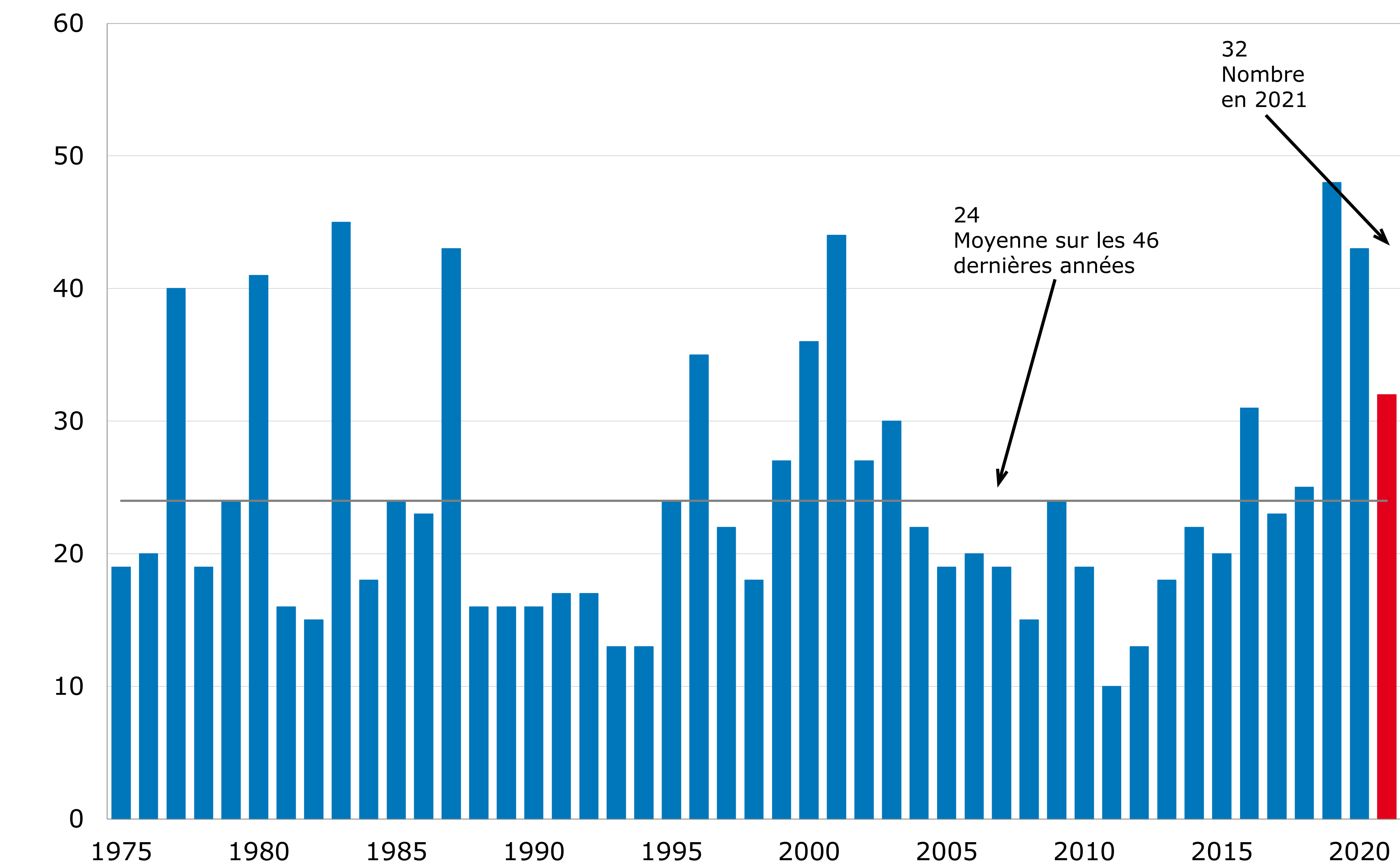
Nombre de séismes de magnitude 2.5 ou plus par an
