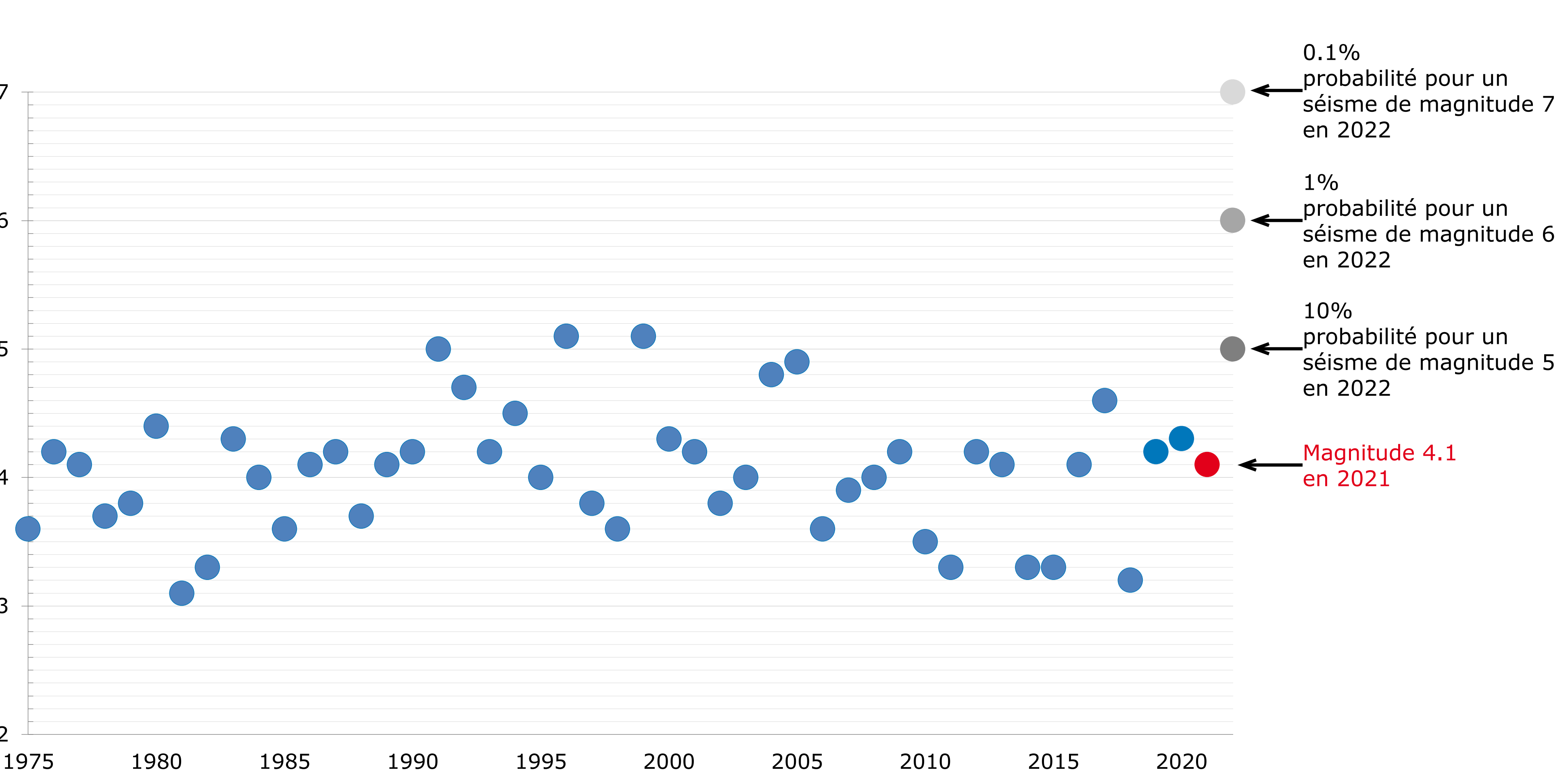
Plus forte magnitude (M) mesurée par an
