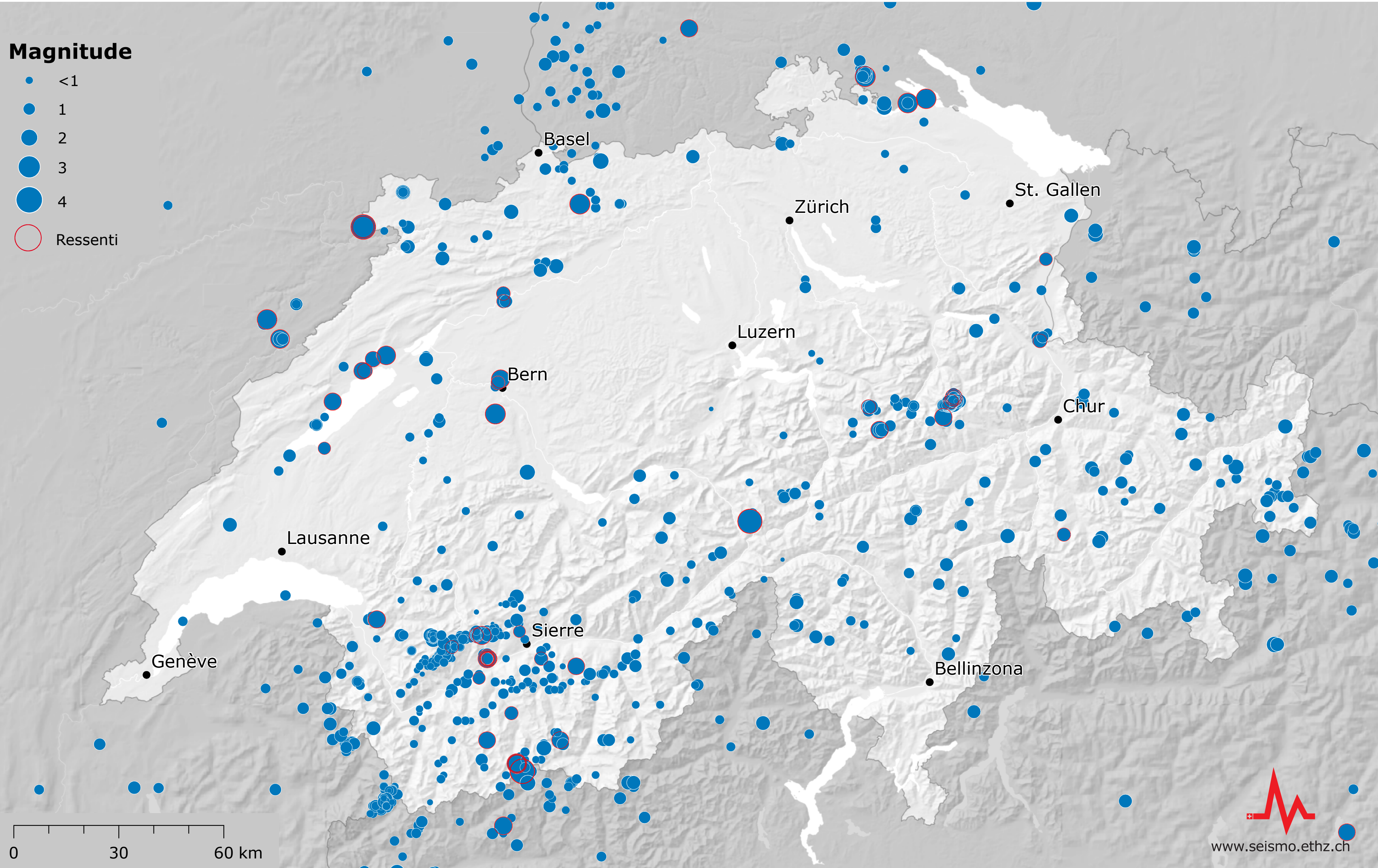
Plus forte magnitude (M) mesurée par an
